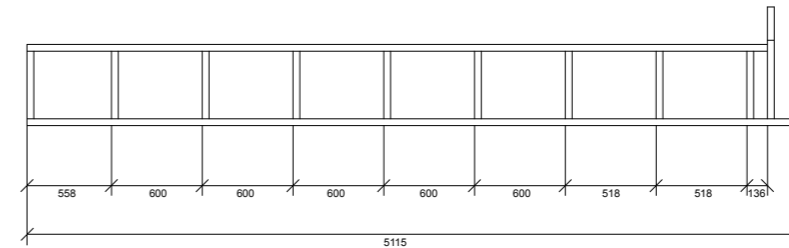
VÄGG ELEVATION - 06
