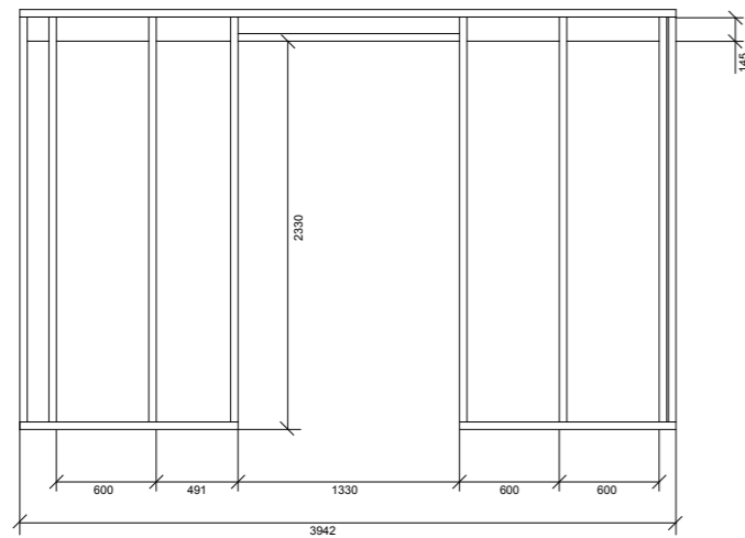
VÄGG ELEVATION - 05
