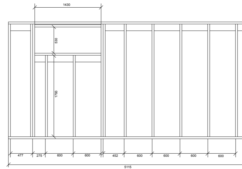
VÄGG ELEVATION - 06
