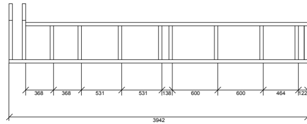
VÄGG ELEVATION - 05
